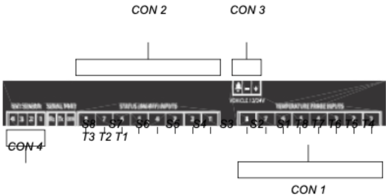
Abbildung 3.2 Schreiberanschlüsse
