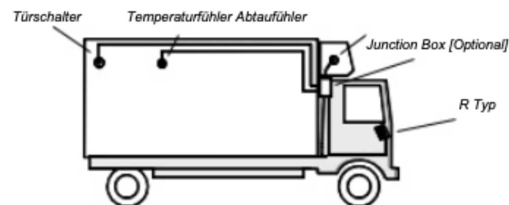
Abbildung 1.2 Interne Montage
