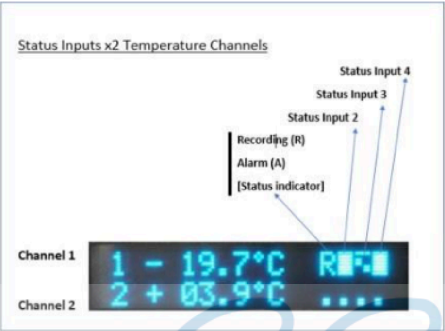
Abbildung 1.4.1 Das Display Status Eingänge x2 Temperaturkanäle
